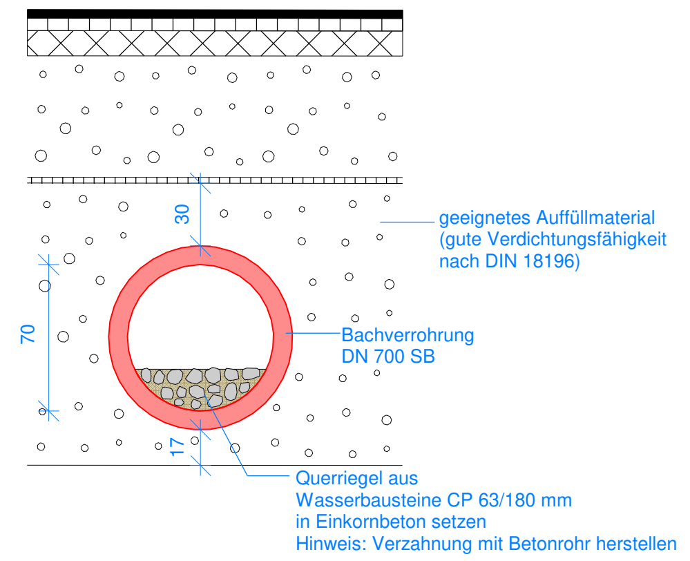
Querschnitt Maßstab 1 : 25
